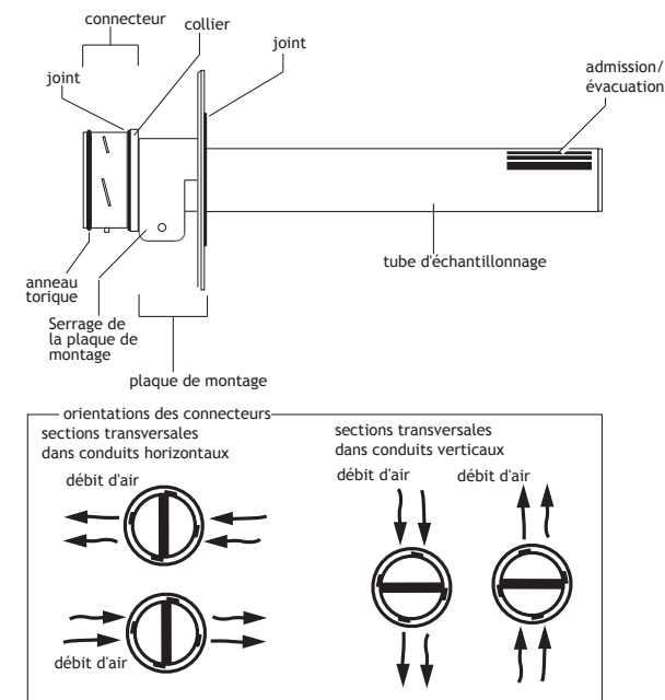
Figure 4: tube d'échantillonnage et plaque de montage
