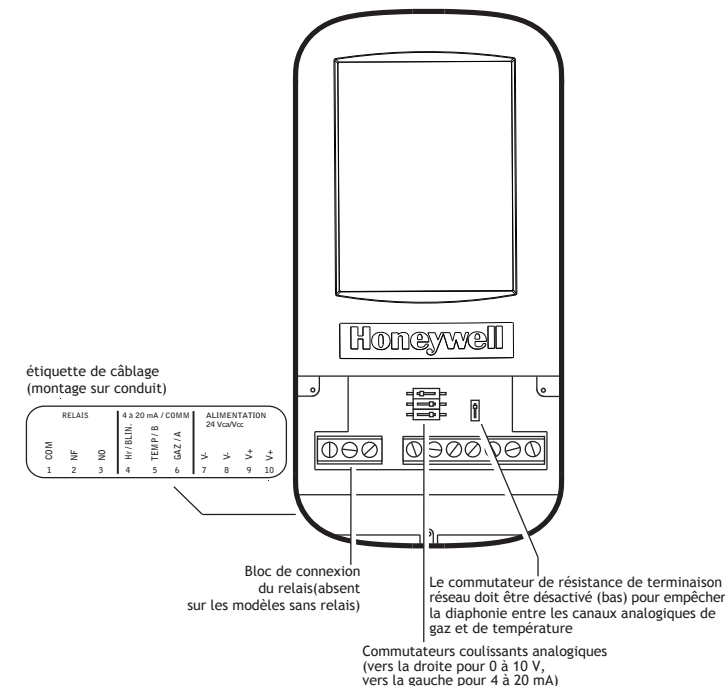
Figure 3: câblage du moniteur monté sur conduit
