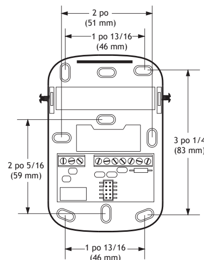
Figure 1: Distances entre les trous de montage sur la plaque arrière (9 trous)
